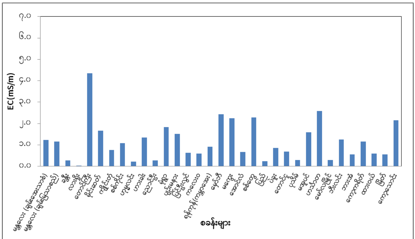
၂၀၂၅ ခုနှစ်၊ အောက်တိုဘာလအတွင်း စခန်း ၃၃ စခန်းတို့၌ ရွာသွန်းခဲ့သောမိုးရေနမူနာများ၏ EC(mS/m) တန်ဖိုးပြပုံ
