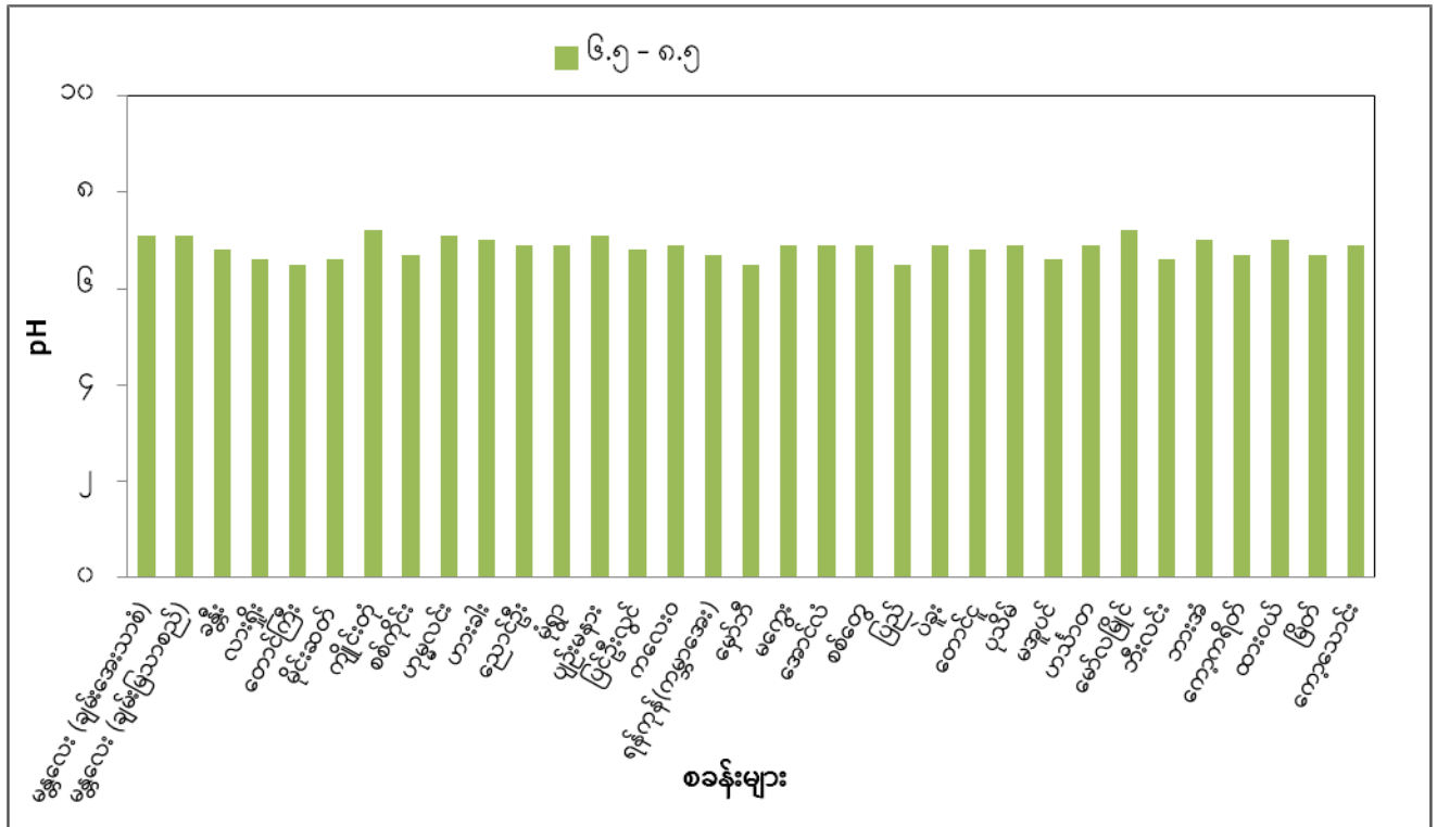
၂၀၂၅ ခုနှစ်၊ အောက်တိုဘာလအတွင်း စခန်း ၃၃ စခန်းတို့၌ ရွာသွန်းခဲ့သော မိုးရေနမူနာများ၏ pH တန်ဖိုးပြပုံ
