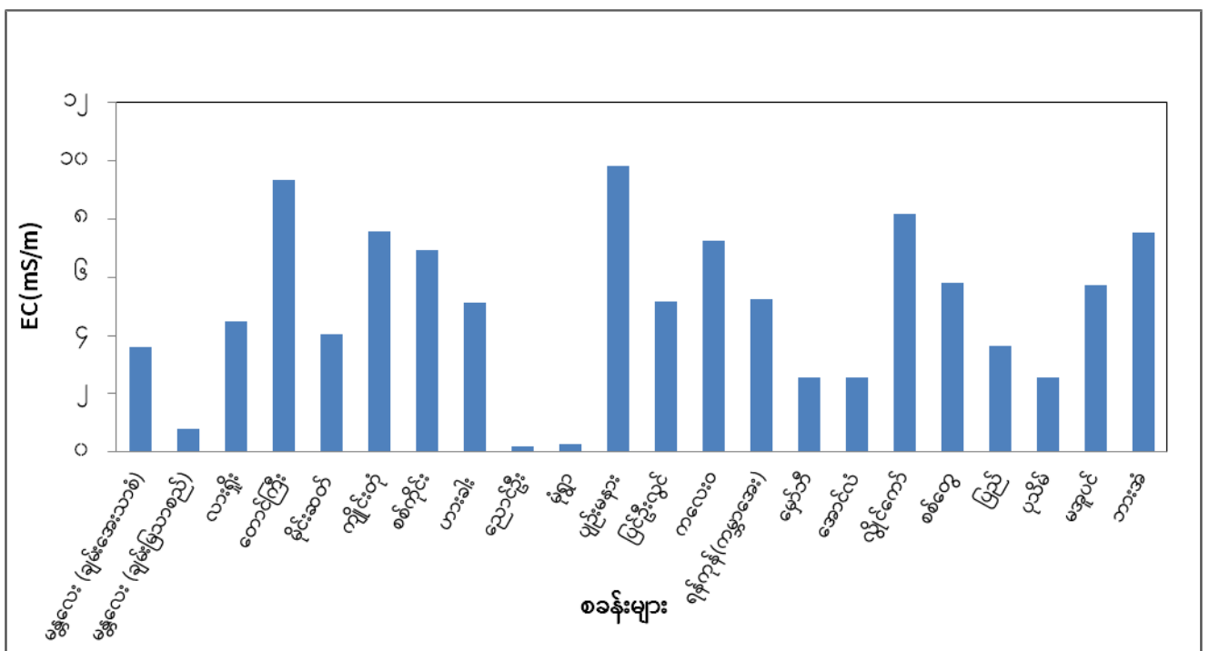
၂၀၂၆ ခုနှစ်၊ မတ်လအတွင်း စခန်း ၂၂ စခန်းတို့၌ ရွာသွန်းခဲ့သော မိုးရေနမူနာများ၏ EC(mS/m) တန်ဖိုးပြပုံ
