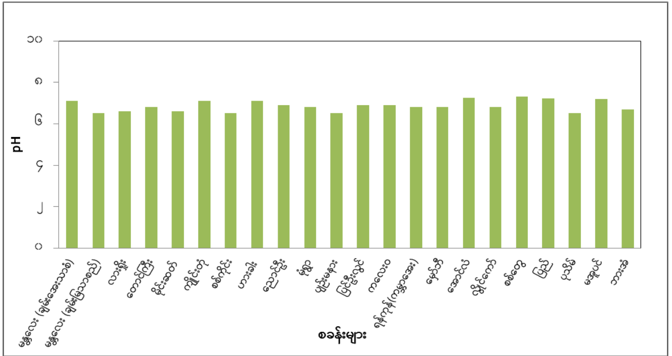
၂၀၂၆ ခုနှစ်၊ မတ်လအတွင်း စခန်း ၂၂ စခန်းတို့၌ ရွာသွန်းခဲ့သော မိုးရေနမူနာများ၏ pH တန်ဖိုးပြပုံ
