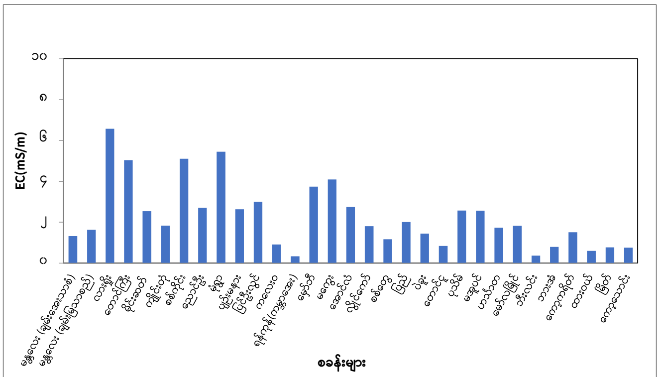
၂၀၂၆ ခုနှစ်၊ ဩဂုတ်လအတွင်း စခန်း ၃၁ စခန်းတို့၌ ရွာသွန်းခဲ့သော မိုးရေနမူနာများ၏ EC(mS/m) တန်ဖိုးပြပုံ
